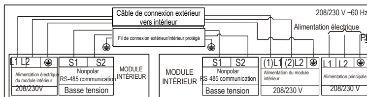
Schéma de connexion (36 K/48K)
