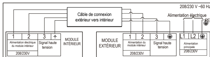
Schéma de connexion (6K/ 1 9 K/1 2 K/ 8K)
