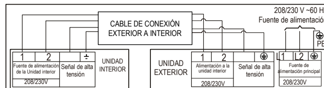
Diagrama de conexión (9K/12K/18K/24K)
